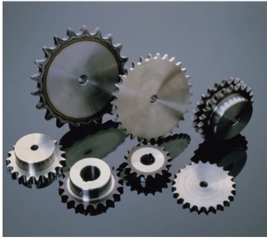
膨大なバリエーションを誇る『標準スプロケット』と、高精度高品質の『FBN スプロケット』
